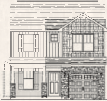
Elevation 5
