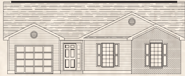
Elevation 3
