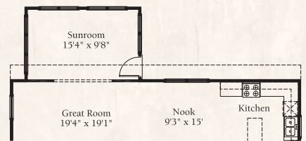
Optional Sunroom
