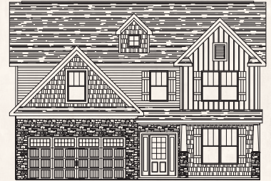
Elevation 6
