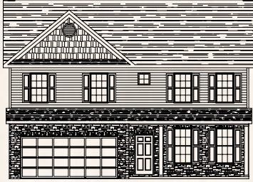
Elevation 4
